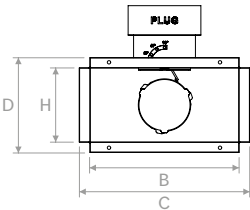
Ansicht von oben | Top view
