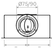
Ansicht von oben | Top view
