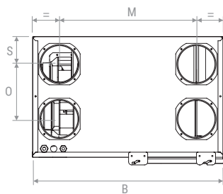
Draufsicht | Top view
