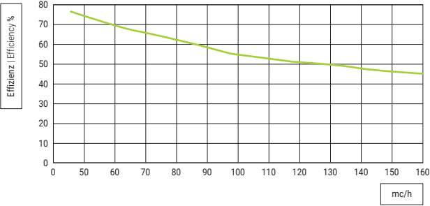
Latentes Effizienz-Diagramm Sommer Außenluft: 35 °C - 57 % R.F. Raumluft: 25 °C - 50 % R.F. Summer latent efficiency chart Fresh air: 35 °C - 57 % R.H. Return air: 25 °C - 50 % R.H.
