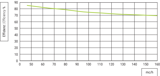
Sensibles Effizienz-Diagramm Sommer Außenluft: 35 °C Raumluft: 25 °C Summer sensible efficiency chart Fresh air: 35 °C Return air: 25 °C
