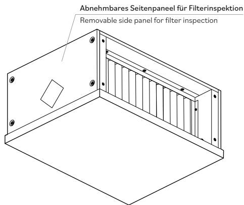
Ansicht von unten | Bottom View
