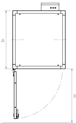
Ansicht von oben | Top view
