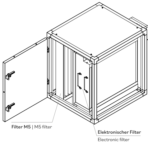
Rückansicht | Rear view
