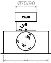
Vista superiore | Top view
