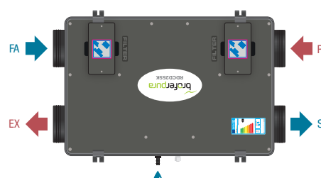
Tipo | Type B1
