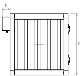
Vista frontale | Top view
