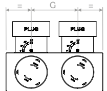
Vue supérieure | Top view
