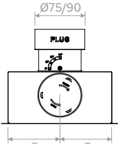
Vue supérieure | Top view
