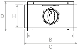
Vue supérieure | Top view
