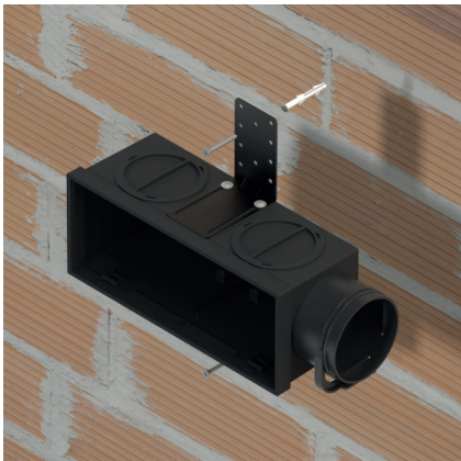
Fissaggio plenum | Plenum box fixing
