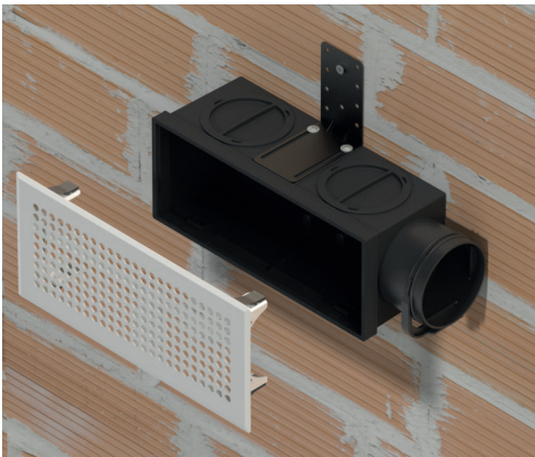
Installazione griglia | Grille installation
