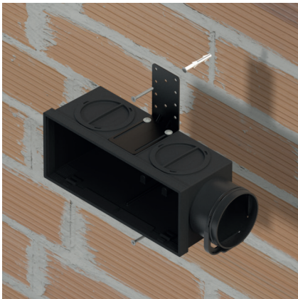
Fissaggio plenum | Plenum box fixing
