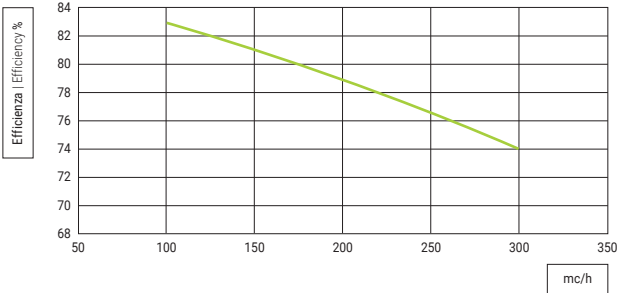
Diagramma efficienza sensibile estiva Aria esterna: 35 °C Aria ambiente: 25 °C Summer sensible efficiency chart Fresh air: 35 °C Return air: 25 °C
