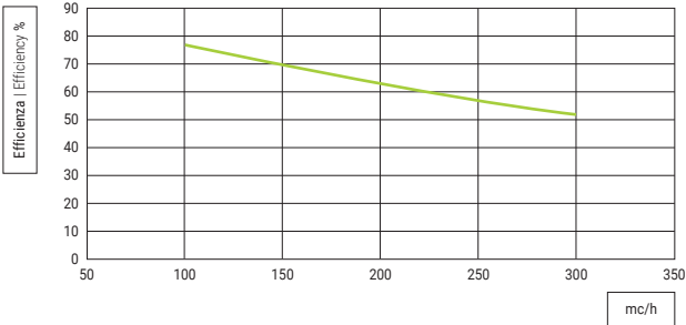
Diagramma efficienza latente estiva Aria esterna: 35 °C - 57 % U.R. Aria ambiente: 25 °C - 50 % U.R. Summer latent efficiency chart Fresh air: 35 °C - 57 % R.H. Return air: 25 °C - 50 % R.H.
