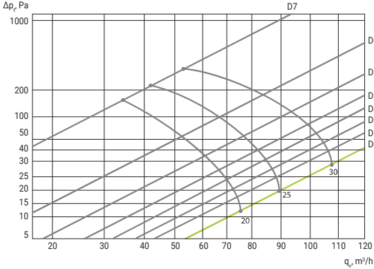
BPDQ 125 RIPRESA ARIA | RETURN AIR
