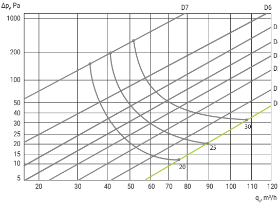
BPDQ 125 MANDATA ARIA | SUPPLY AIR
