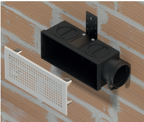
Installazione griglia | Grille installation
