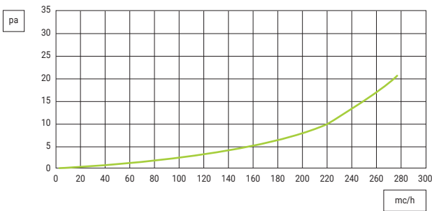
PLUGPVMCMR PERDITE DI CARICO PER SINGOLO FLUSSO | AIR PRESSURE DROP FOR SINGLE
