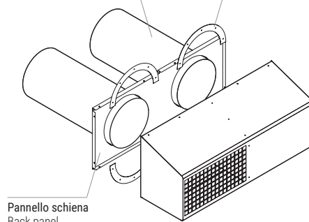
Canali di uscita del muro Ducts coming out of the wall
