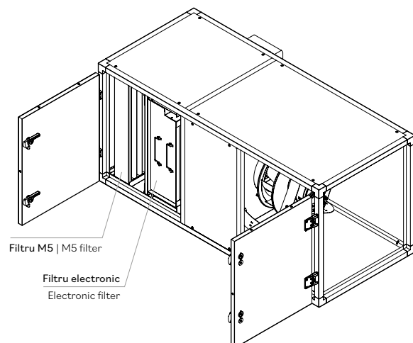
Vedere din spate | Rear view
