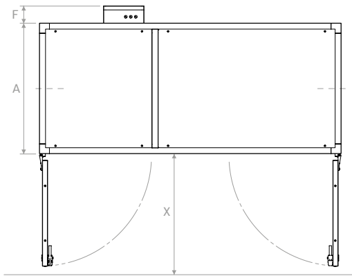
Vedere de sus | Top view
