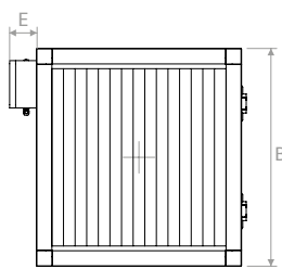
Vedere de sus | Top view
