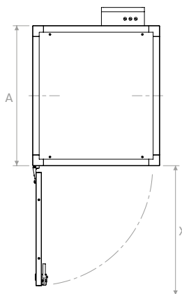
Vedere de sus | Top view
