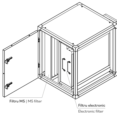
Vedere din spate | Rear view
