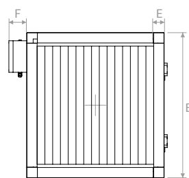
Vedere din față | Front view
